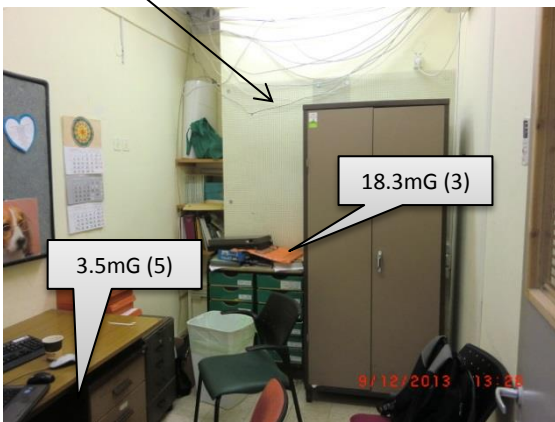
תמונה 3 : משרד רכז טיולים – קיר גב לוח החשמל
