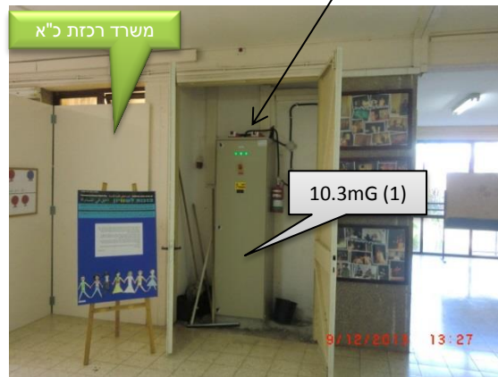
תמונה 2 : לוח החשמל במבואת הכניסה לבניין
